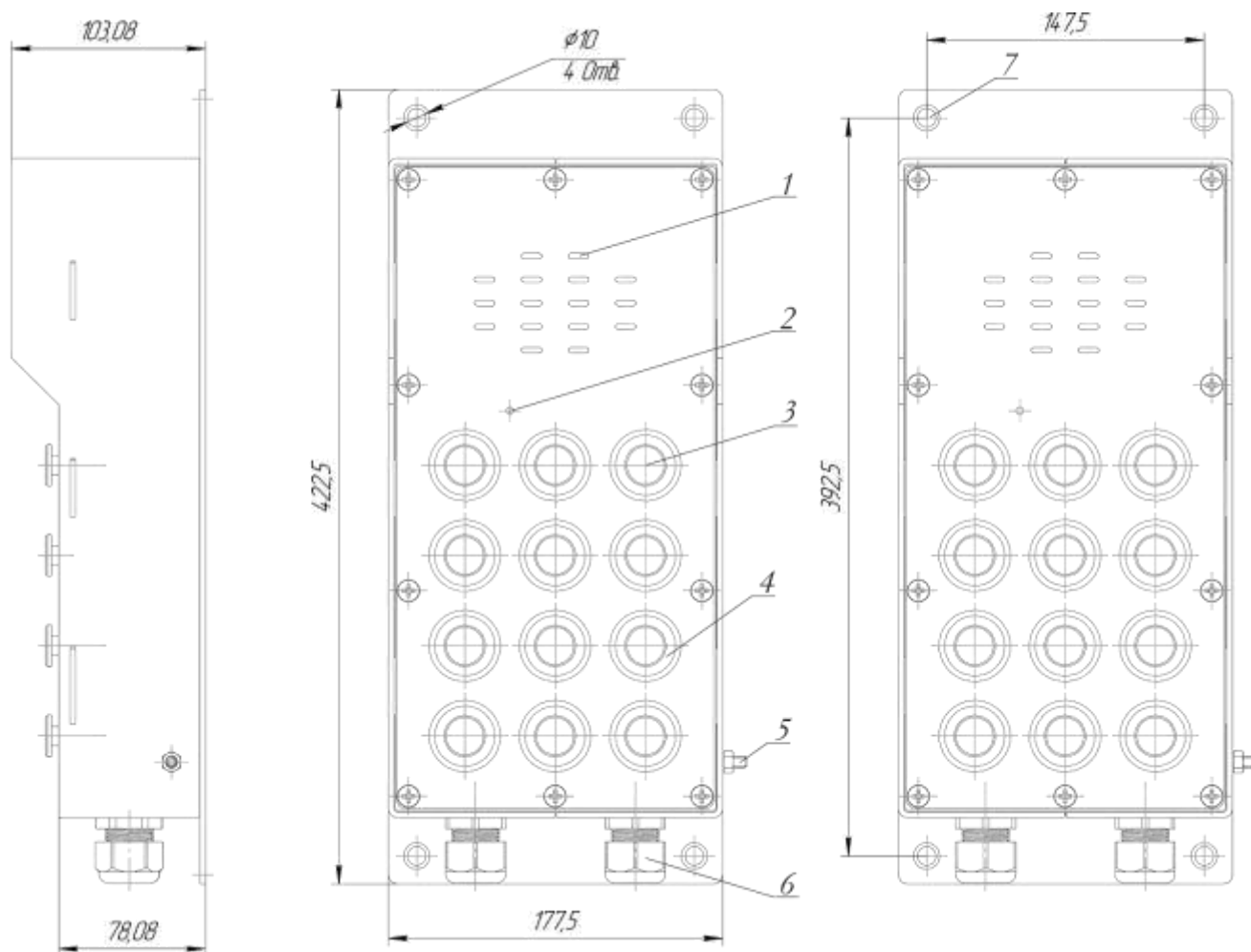
Рисунок 2 – Внешний вид УПГ-38Е, где
