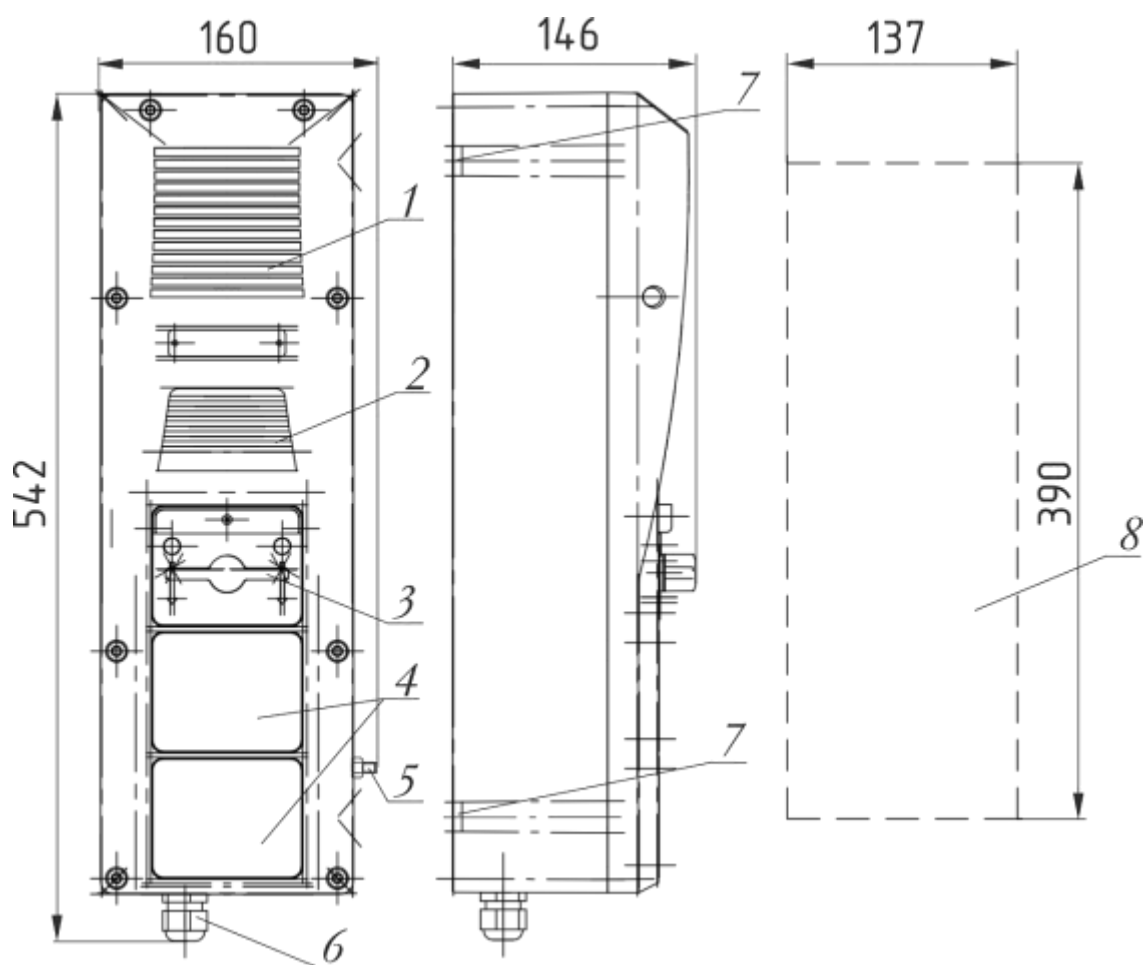
Рисунок 2 – Внешний вид УПГ-ЕхМ-Е-Исп.78
